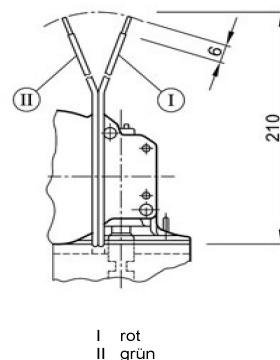
Anschluss K178
