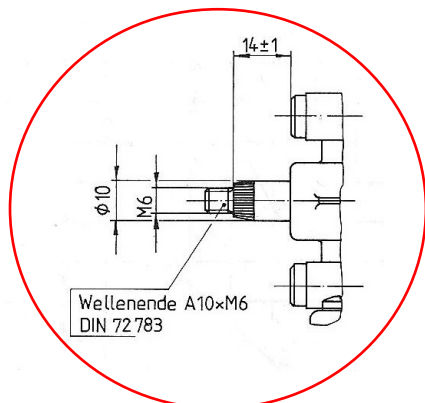
Abtriebswelle W63
