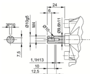
Abtriebswelle W304
