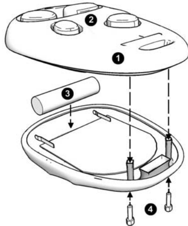
■ Fernbedienung PULT 6204 durch 1 Batterie 27A 12V gespeist
