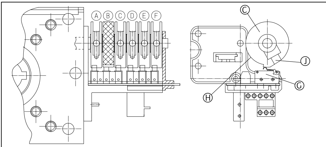
Abb. 13: Referenzpunkteinstellung
