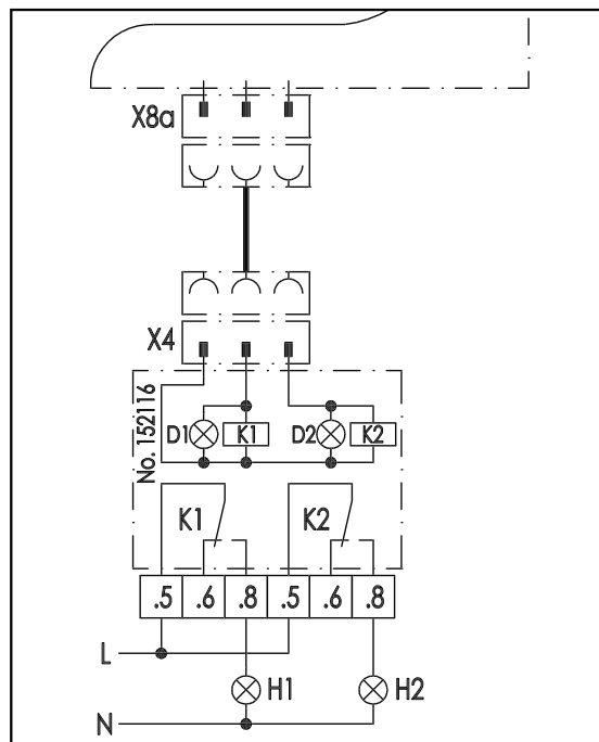
Abb. 21: Schaltplan
