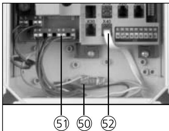
Abb. 7: Anschlüsse in der Steuerung Control 145N
