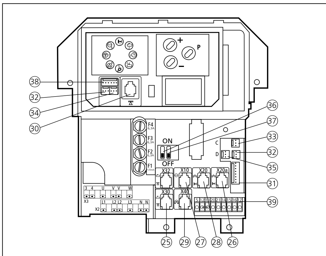
Abb.4: Anschlüsse der Steuerung
