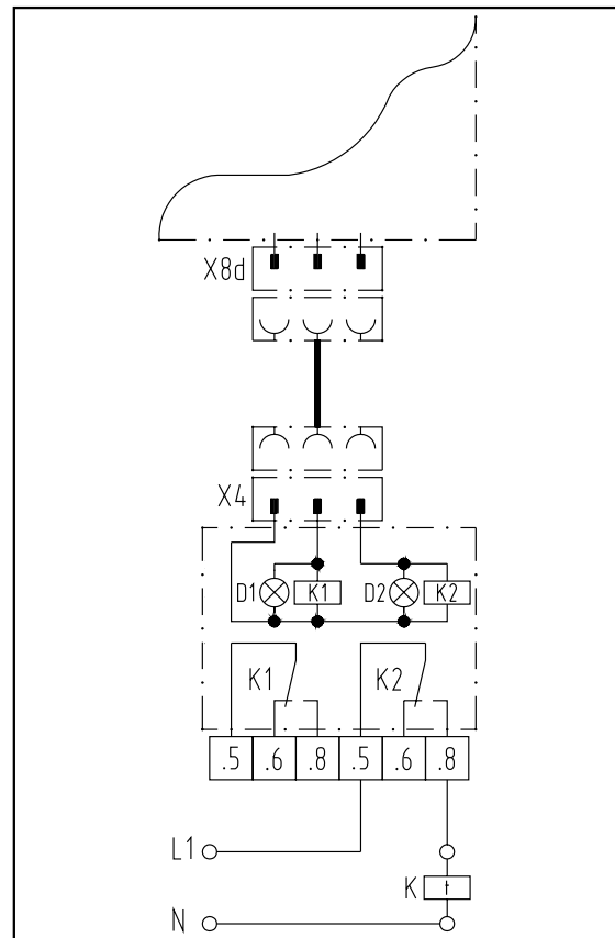
Abb. 24: Schaltplan
