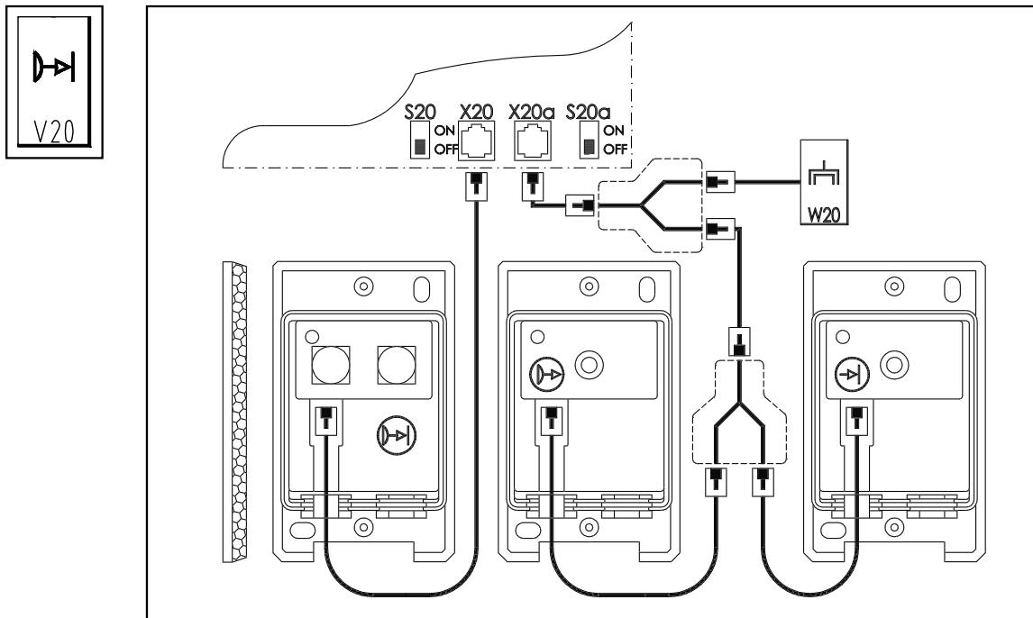
Abb. 19: Schaltplan
