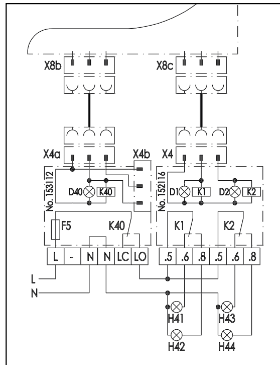
Abb. 23: Schaltplan
