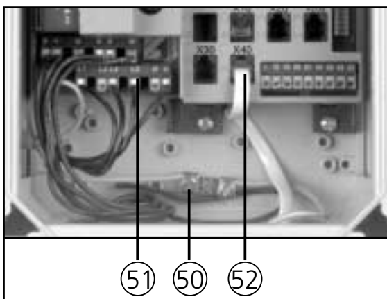
Abb. 5: Anschlüsse in der Steuerung Control 144N
