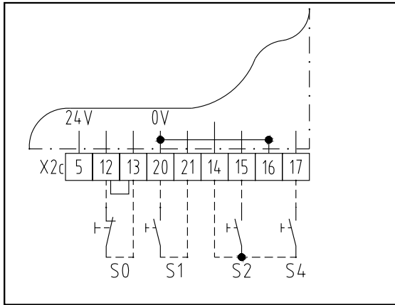
Abb. 17: Schaltplan
