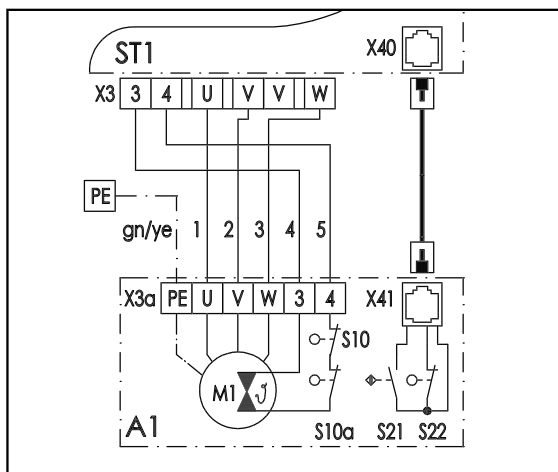
Abb. 6: Schaltplan mit Steuerung Control 144N
