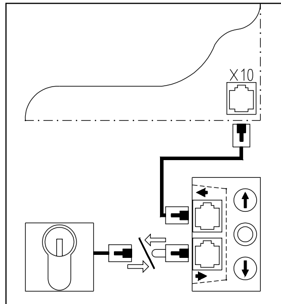
Abb. 14: Schaltplan
