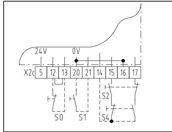
Abb. 18: Schaltplan
