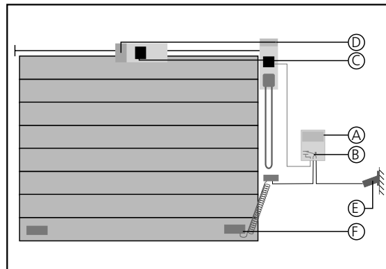
Abb.1: Übersichtsskizze der Torumgebung
