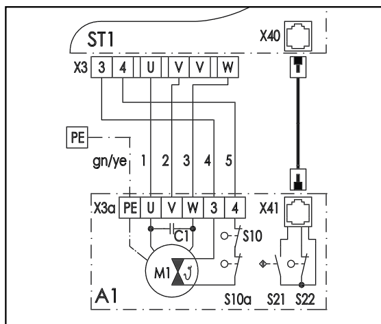
Abb. 8: Schaltplan mit Steuerung Control 145N
