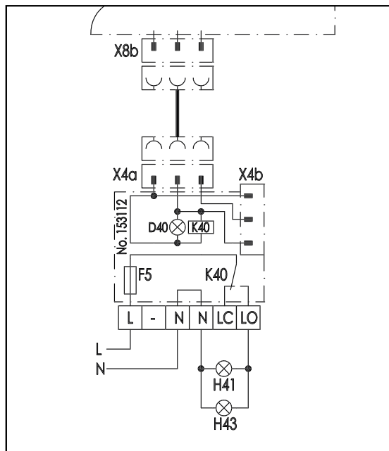
Abb. 22: Schaltplan
