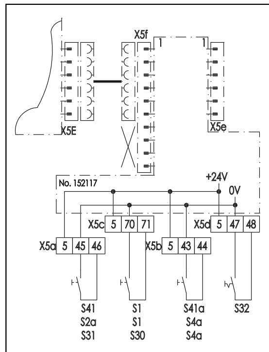
Abb. 20: Schaltplan
