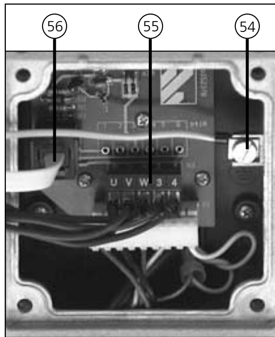
Abb. 9: Anschlüsse im Torantrieb
