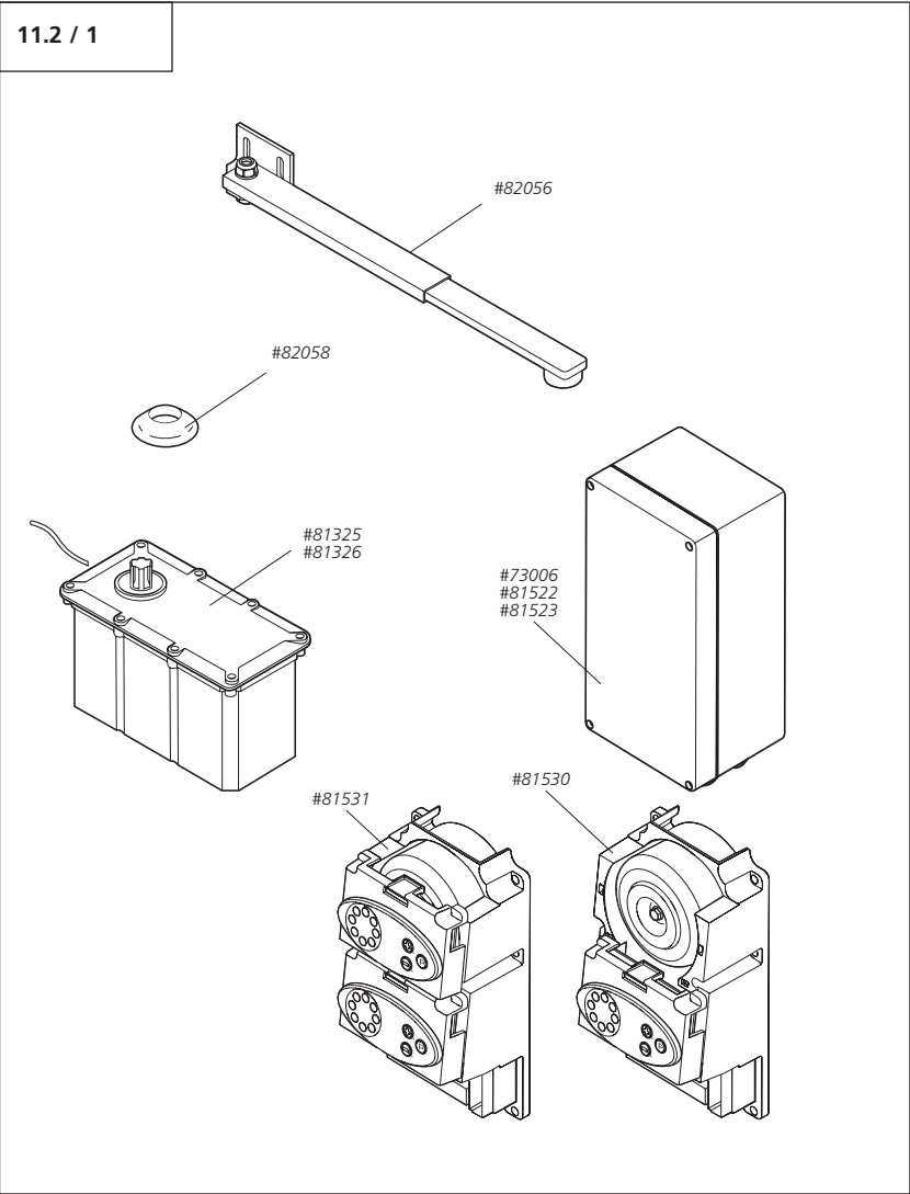
Legende Ersatzteile 11.2 / 1
