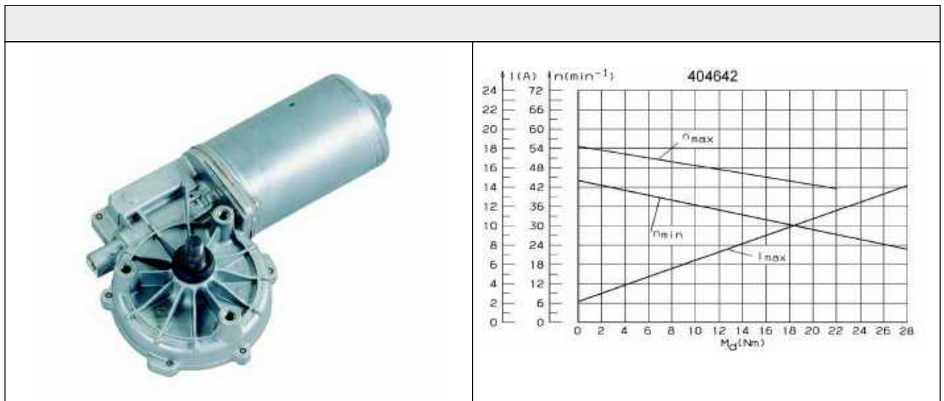
Abtriebswelle W404642
